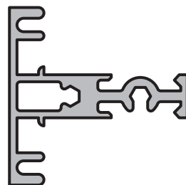
TRAVESAÑO VIDRIO REPARTIDO Perfil: M-2665 Peso: 0,562 Kg/m Matriz: M2665
