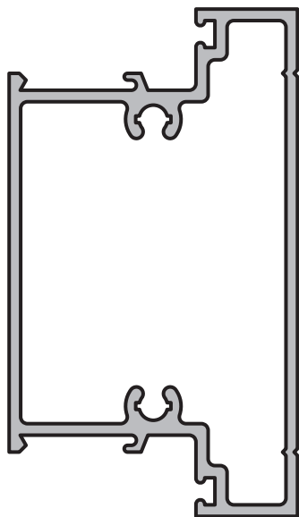
TRAVESAÑO Perfil: 5617 Peso: 1,277 Kg/m
