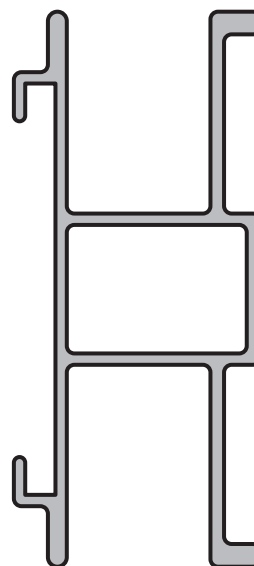
GUÍA CENTRAL - CORTINA COMUN
