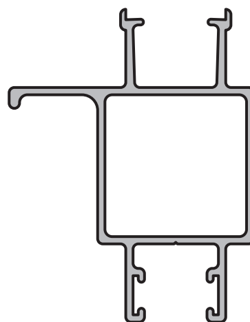
PARANTE LATERAL REFORZADO - PUERTA CORREDIZA Perfil: 220 Peso: 0,821 Kg/m Matriz: M2673
