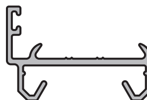
MARCO ANGOSTO - PUERTA CON BISAGRA ENCOLIZADA /POSTIGON Perfil: 508 Peso: 0,394 Kg/m Matriz: M1542
