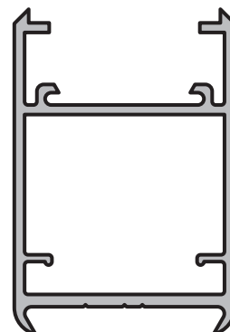
BATIENTE DE HOJA Perfil: 174 Peso: 0,713 Kg/m Matriz: M2260
