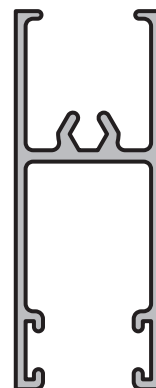
ZOCALO Y CABEZAL - HOJA CORREDIZA
