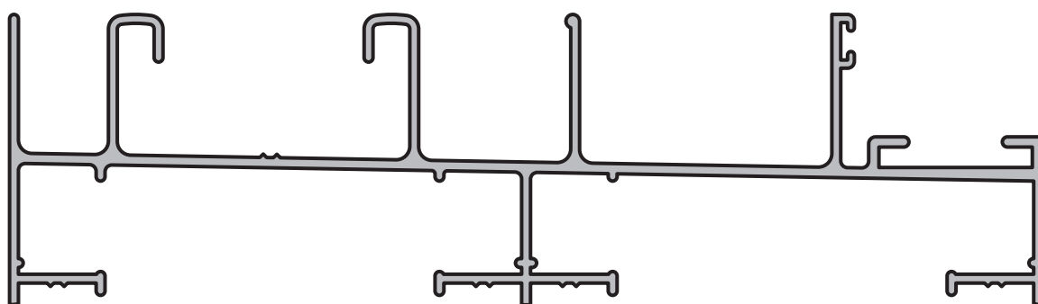
MARCO UNIFICADO CON POSTIGON DE REBATIR
