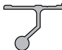
BISAGRA Perfil: 215 Peso: 0,338 Kg/m Matriz: M2704
