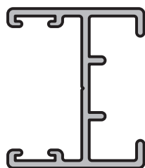
CIERRE CENTRAL - PUERTA Y VENTANA CORREDIZA 4 HOJAS Perfil: 19 Peso: 0,389 Kg/m Matriz: M0686
