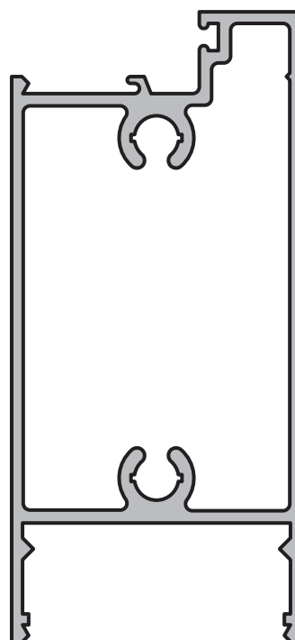
ZOCALO Perfil: 5624 Peso: 1,569 Kg/m
