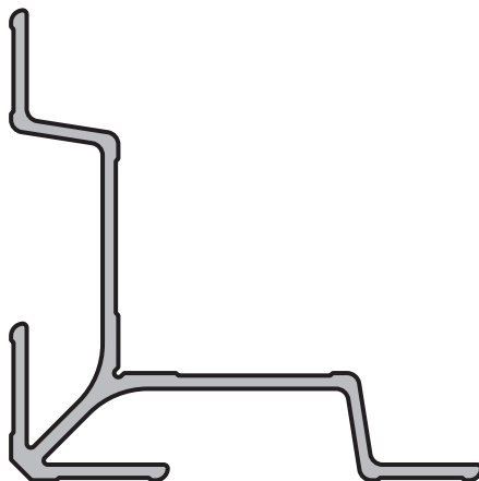
ESCUADRA DE ARMADO PARTE A B y C Perfil: 37 Peso: 0,745 Kg/m Matriz: M0642
