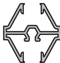
TRAVESAÑO VIDRIO REPARTIDO Perfil: 6571 Peso: 0,359 Kg/m
