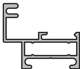
POSTIGO Perfil: M-2562 Peso: 0,419 Kg/m Matriz: M2562
