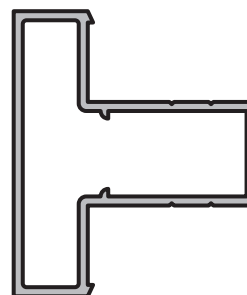
TRAVESAÑO ANGOSTO Perfil: 528 Peso: 0,443 Kg/m Matriz: M2530
