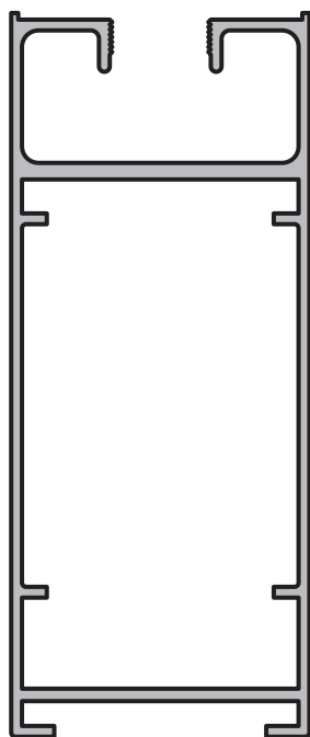
PARANTE Perfil: 3938 Peso: 1,120 Kg/m
