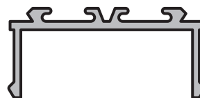
PORTACONTRAVIDRIO/ PORTAFELPA Perfil: 5628 Peso: 0,289 Kg/m
