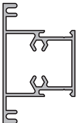
TRAVESAÑO ANGOSTO Perfil: M-2211 Peso: 0,783 Kg/m Matriz: M2211
