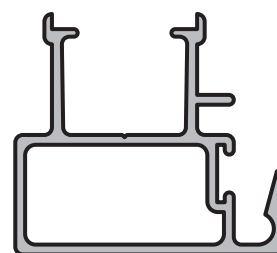
PARANTE CENTRAL - HOJA CORREDIZA
