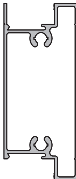
TRAVESAÑO / ZOCALO / CABEZAL HOJA Perfil: 3941 Peso: 1,039 Kg/m
