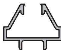
BASTIDOR VIDRIO REPARTIDO CORREDIZA Perfil: 6572 Peso: 0,243 Kg/m
