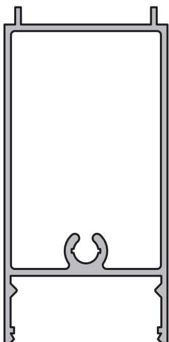
COMPLEMENTO ZOCALO Perfil: 5623 Peso: 1,293 Kg/m
