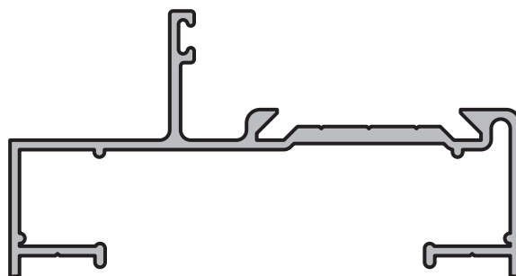
MARCO Perfil: 211 Peso: 0,780 Kg/m Matriz: M2699
