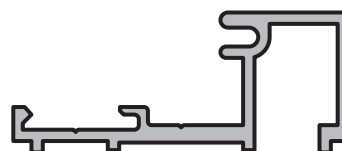
PORTA CONTRAVIDRIOS Perfil: 43 Peso: 0,429 Kg/m Matriz: M0844
