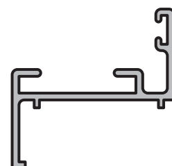
MARCO POSTIGO Perfil: 6336 Peso: 0,300 Kg/m
