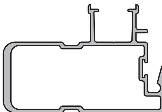
PARANTE CENTRAL REFORZADO - PUERTA CORREDIZA Perfil: 204 Peso: 1,112 Kg/m Matriz: M2632
