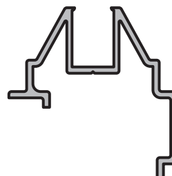
BASTIDOR VIDRIO REPARTIDO PAÑO FIJO Perfil: 6765 Peso: 0,316 Kg/m
