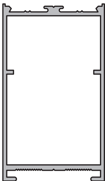
HOJA Perfil: 5616 Peso: 1,288 Kg/m
