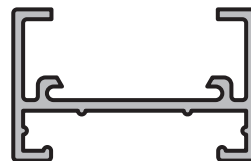
SOPORTE TABLILLA DE POSTIGON Perfil: 148 Peso: 0,340 Kg/m Matriz: M1986
