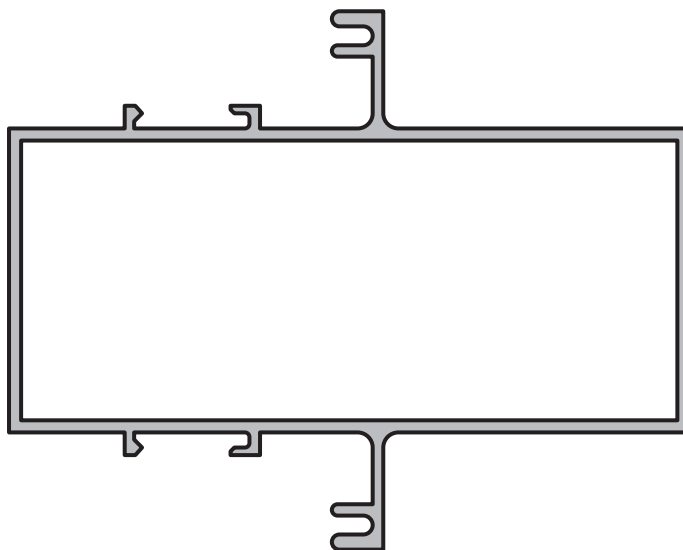
TRAVESAÑO PAÑO FIJO TUBULAR 90 x 40 mm.
