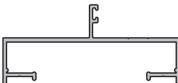
MARCO - PUERTA PLACA SIMPLE CONTACTO
