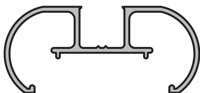
PORTA PLACA REDONDO Perfil: 6486 Peso: 0,467 Kg/m
