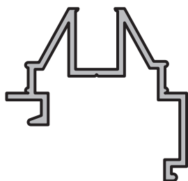
BASTIDOR VIDRIO REPARTIDO PAÑO FIJO Perfil: 802 Peso: 0,389 Kg/m Matriz: M2776
