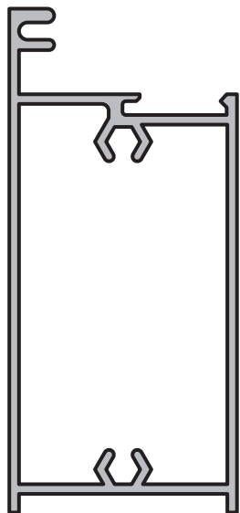
ZOCALO MEDIANO Perfil: M-2809 Peso: 0,896 Kg/m Matriz: M2809
