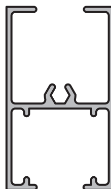
TRAVESAÑO POSTIGON DE ABRIR PARA 5800 Perfil: 226 Peso: 0,591 Kg/m Matriz: M2806
