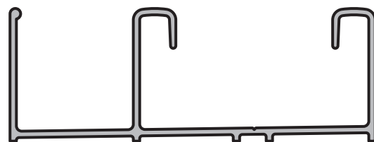
GUIA CORREDIZA CON MOSQUITERO Perfil: 6568 Peso: 0,540 Kg/m
