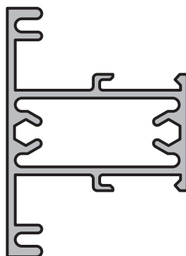
TRAVESAÑO CHICO - PAÑO FIJO Perfil: 687 Peso: 0,745 Kg/m Matriz: M1777
