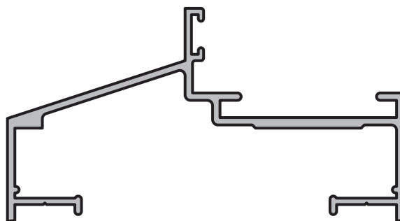
MARCO Perfil: 3939 Peso: 0,715 Kg/m
