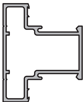
TRAVESAÑO CHICO Perfil: 3937 Peso: 0,505 Kg/m
