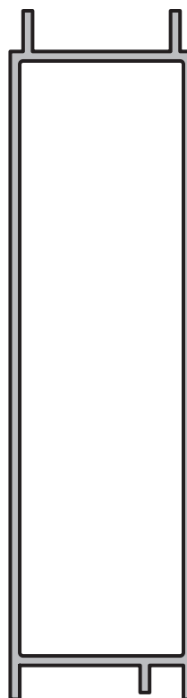
TABLILLA Perfil: 207 Peso: 0,967 Kg/m Matriz: M2695
