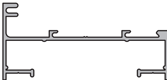
MARCO - PAÑO FIJO (3 a 57 mm.)
