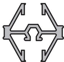
TRAVESAÑO VIDRIO REPARTIDO Perfil: 801 Peso: 0,434 Kg/m Matriz: M2775
