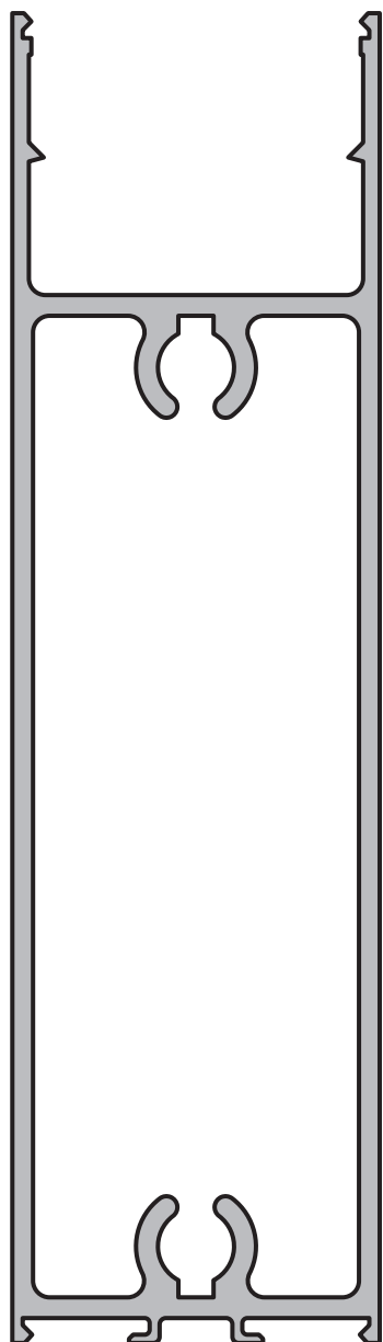
TRAVESAÑO REFORZADO HOJA Perfil: 65 Peso: 3,059 Kg/m Matriz: M0954
