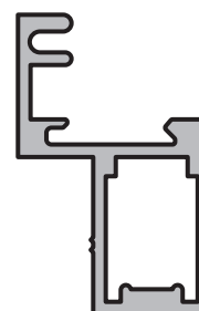
HOJA SECUNDARIA PUERTA Perfil: 136 Peso: 0,497 Kg/m Matriz: M1876
