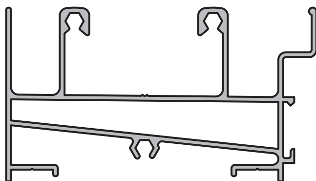
UMBRAL CON CAJA DE AGUA CORREDIZA Perfil: 219 Peso: 1,369 Kg/m Matriz: M2677
