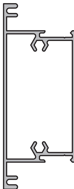
TRAVESAÑO ANCHO Perfil: M-2212 Peso: 1,010 Kg/m Matriz: M2212
