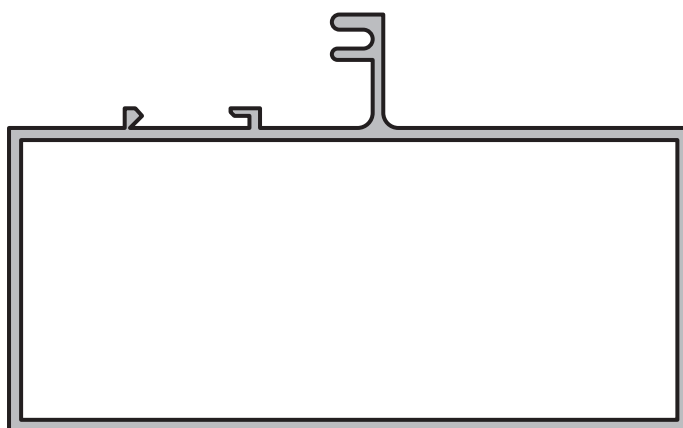
PAÑO FIJO TUBULAR 90 x 40 mm.
