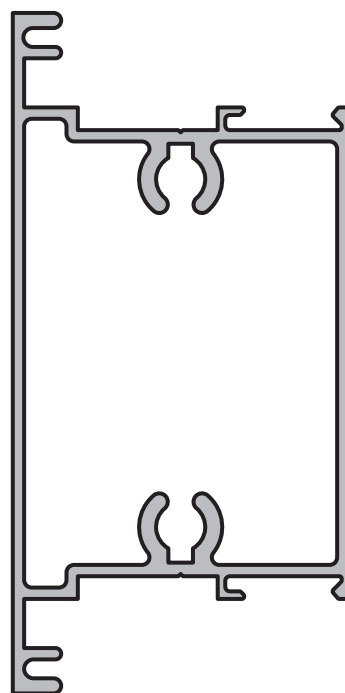
TRAVESAÑO INTERMEDIO
