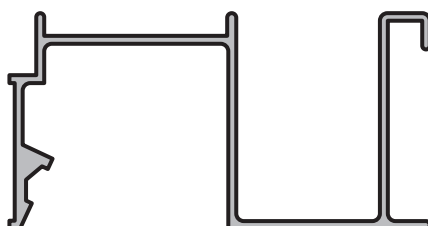
GUÍA CORTINA DE ENROLLAR
