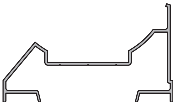
PERFIL ROTULA
