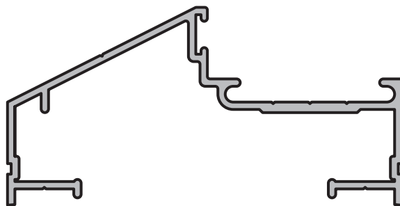
MARCO Perfil: M-2473 Peso: 0,724 Kg/m Matriz: M2473
