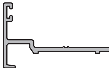
DOBLE CONTACTO Perfil: 5622 Peso: 0,418 Kg/m
