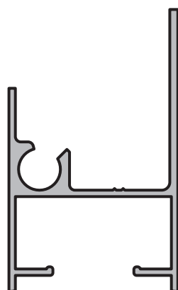
MARCO 31,5 mm. Perfil: 6565 Peso: 0,556 Kg/m Matriz: P6565
