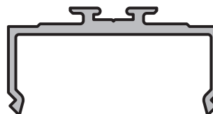
PORTA BURLETE Y PORTA CONTRAVIDRIO Perfil: 23 Peso: 0,394 Kg/m Matriz: M0692
