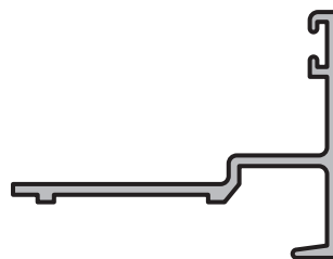
DOBLE CONTACTO Perfil: 3940 Peso: 0,284 Kg/m
