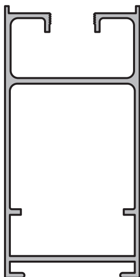
PARANTE MEDIANO Perfil: 3792 Peso: 0,961 Kg/m
