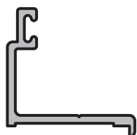
MARCO HOJA SECUNDARIA Perfil: 525 Peso: 0,213 Kg/m Matriz: M2335
