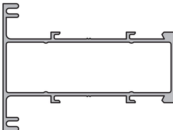
TRAVESAÑO - PAÑO FIJO (3 a 57 mm.)
