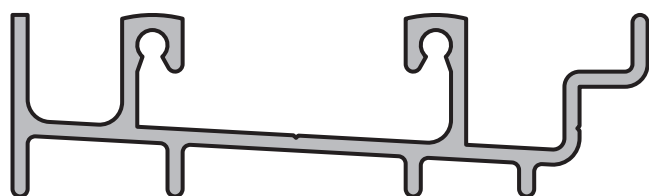
UMBRAL - PUERTA CORREDIZA Perfil: 17 Peso: 1,050 Kg/m Matriz: M0688
