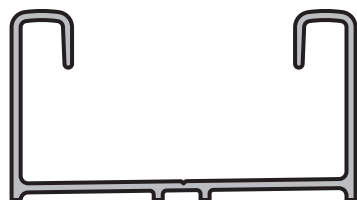
GUIA CORREDIZA SIMPLE Perfil: 6567 Peso: 0,383 Kg/m
