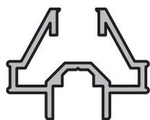
BASTIDOR VIDRIO REPARTIDO CORREDIZA Perfil: 800 Peso: 0,305 Kg/m Matriz: M2774
