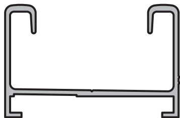
GUIA CON ESCUADRA PARA CORREDIZA Perfil: 690 Peso: 0,489 Kg/m Matriz: M1861
