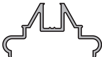
PORTA PLACA RECTO Perfil: 6487 Peso: 0,367 Kg/m
