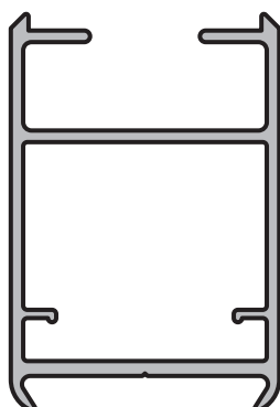
PARANTE POSTIGON DE ABRIR PARA 5800 Perfil: 227 Peso: 0,712 Kg/m Matriz: M2805
