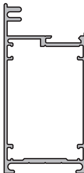
PARANTE MEDIANO Perfil: M-2666 Peso: 0,907 Kg/m Matriz: M2666
