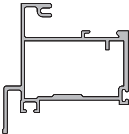
HOJA SIMPLE Perfil: 140 Peso: 1,064 Kg/m Matriz: M1901
