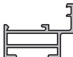
HOJA POSTIGO Perfil: 6335 Peso: 0,370 Kg/m
