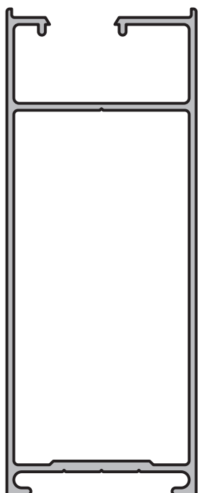
BATIENTE SIN CONTRAVIDRIO Perfil: M-2894 Peso: 1,007 Kg/m Matriz: M2894
